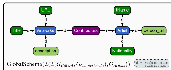
Fig. 20. Generated global schema.
